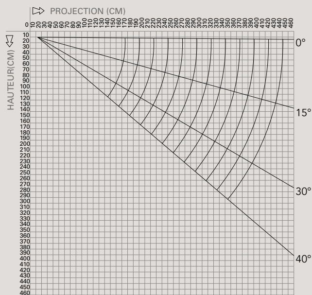
DIAGRAMME D'INCLINAISON
